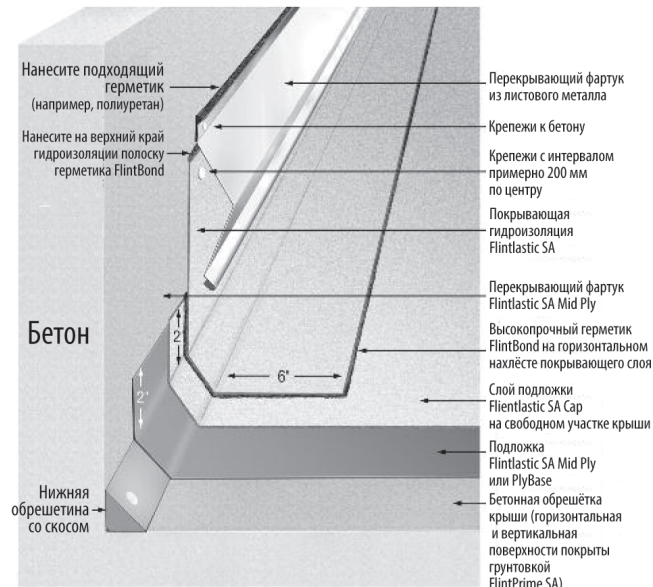
Рис. 5-32. Укладка на бетон в двухслойной системе.
