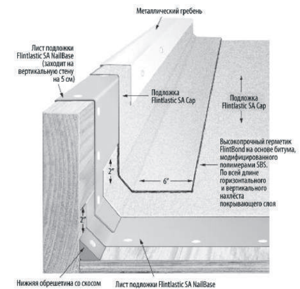
Рис. 5-29. Другой вариант паряпетной стенки в двухслойной системе.
