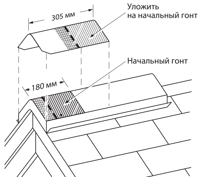
Рис. 12-13. Уложите целый покрывающий гонт на начальный кусок, вровень с его нижними и боковыми краями.
