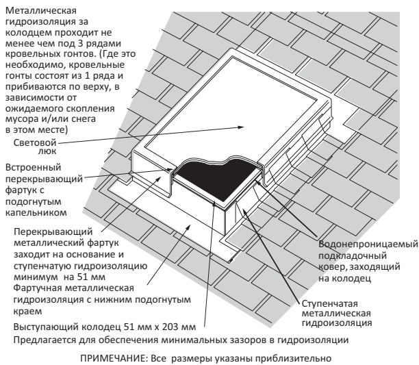
Рис. 6-26: Основные детали из листового металла, используемые со световым люком
