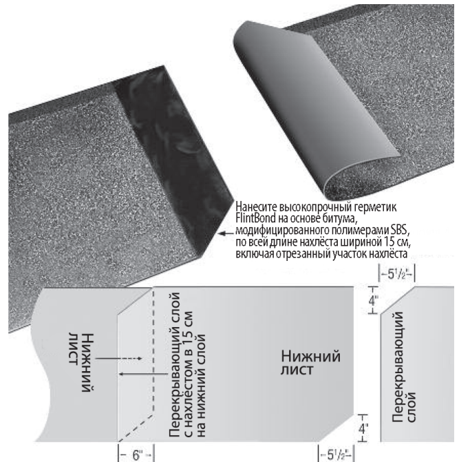
Рис. 5-24. Отрежьте листы нижних и верхних листов, как показано на рисунке.
