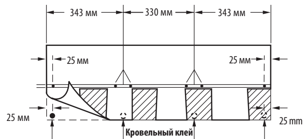
Рис. 12-5. На крутых скатах вбивайте шесть гвоздей и наносите четыре капли битумного кровельного клея.
