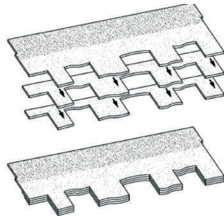
Рис. 2-7: Конструкция гонта Presidential TL.
