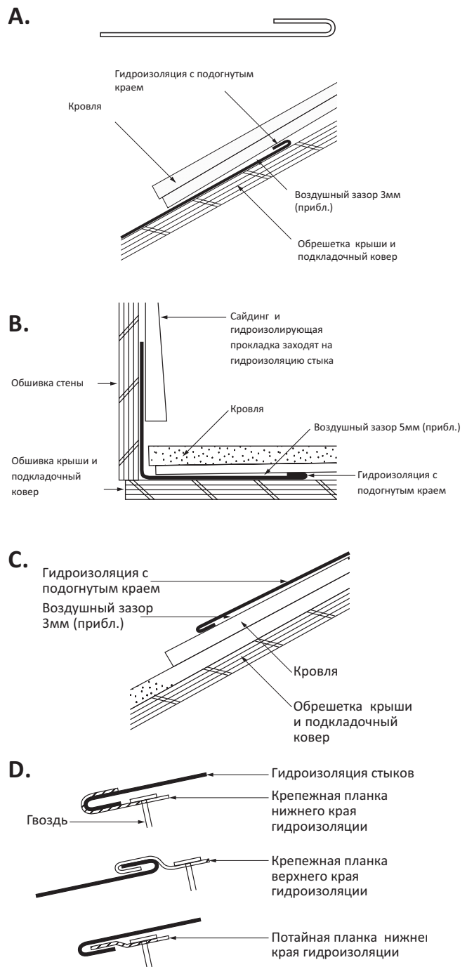
Рис. 6-27: Подогнутый край – очень важная деталь гидроизоляции крыши.
