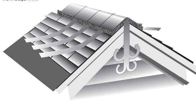
Рис. 7-22. Вентиляционный конек с внутренней перегородкой или вообще без перегородки не «вытягивает» воздух из чердачного помещения через обе стороны вентилярующей секции.
