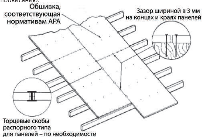
Рис. 4-1: Правильный монтаж обшивки, соответствующей нормативам APA, для укладки кровли.
