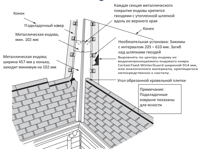
Рис. 6-20: Типичная закрепленная кляммерами открытая ендова
