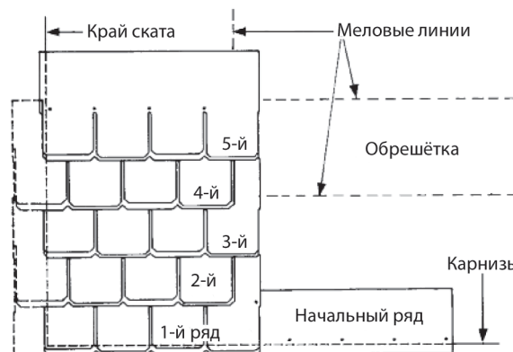
Рис. 16-6. Вертикальный метод укладки.
