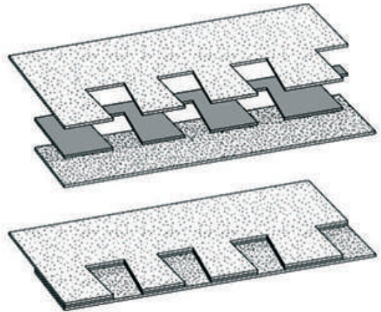
Рис. 2-6: Конструкция гонта Landmark TL.
