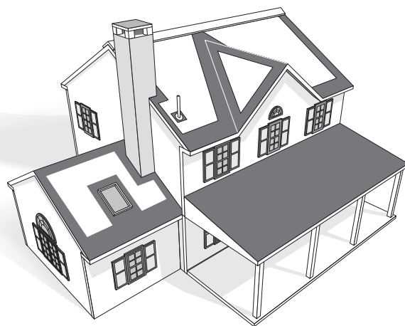
Рис. 7-6. Области, окрашенные темным цветом - участки, защищенные системой WinterGuard от проникновения талых вод, образующихся в результате таяния снега и льда.
