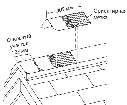
Рис. 13-20. Используйте метки, чтобы выровнять гонты по центру на рёбрах и коньках, а также оставлять открытый участок высотой 12,7 см.
