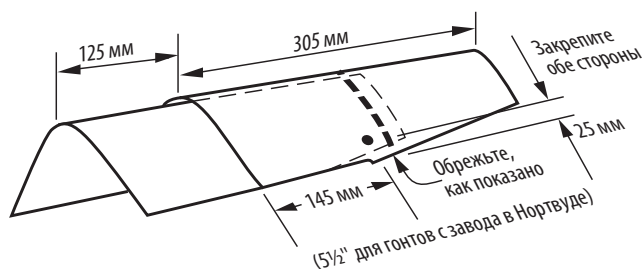
Рис. 10-25. Укладка покрывающих гонтов на рёбра и коньки.
