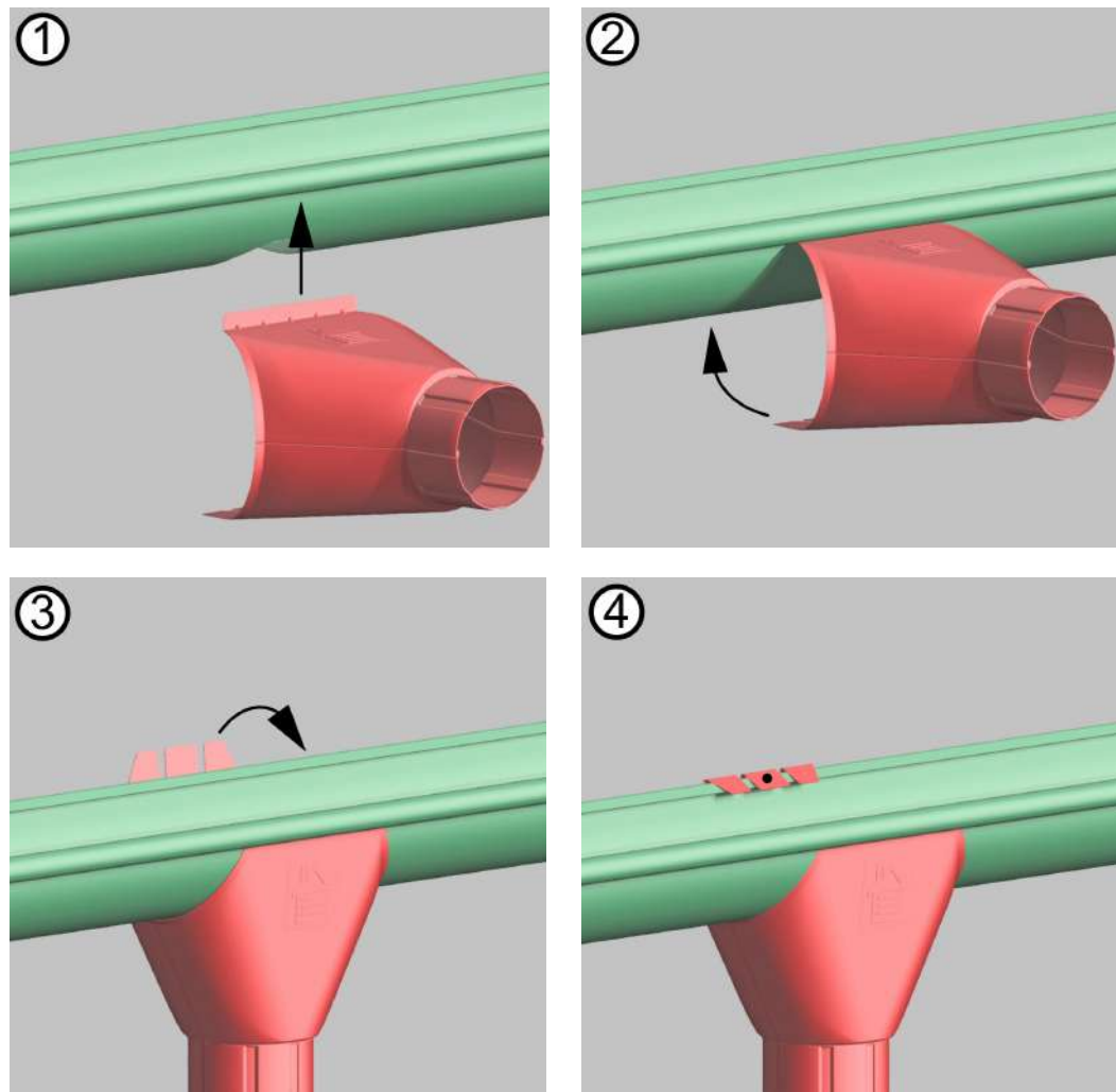
Рис. 14 Установка воронки
