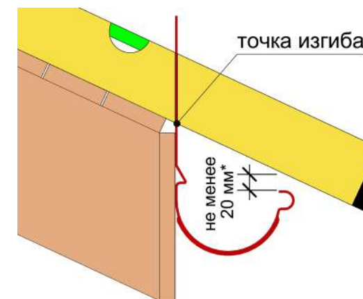
Рис. 3 Нахождение точки изгиба на самом верхнем крюке
