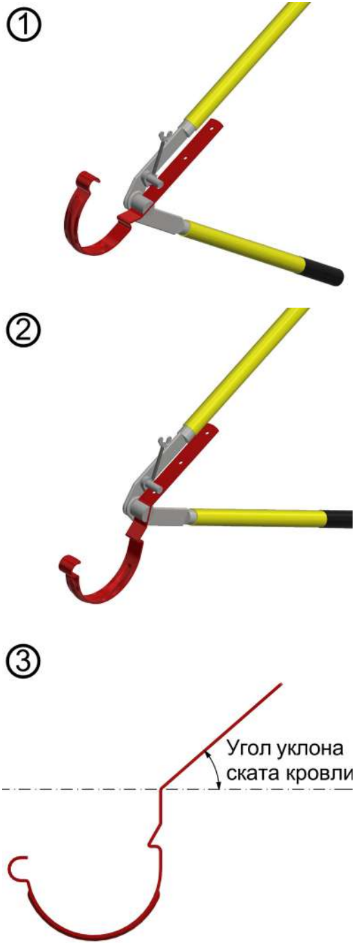
Рис. 5 Загиб карнизного крюка при помощи кронштейногиба
